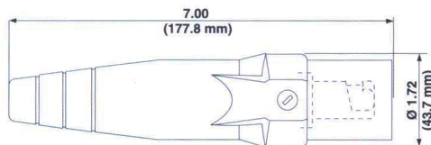
CLAVIJA MACHO SEPARABLE – TORNILLO DE SUJECIÓN DOBLE
