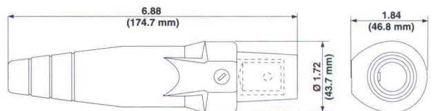
CLAVIJA HEMBRA SEPARABLE – TORNILLO DE SUJECIÓN DOBLE
